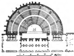
Grundriss eines griechischen Theaters.
